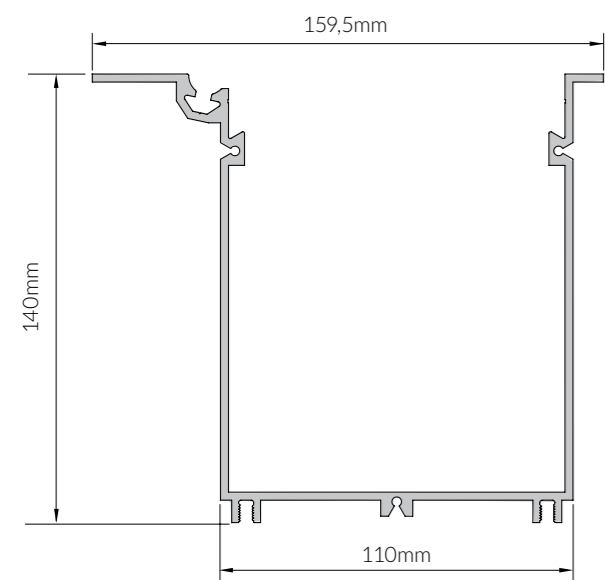
Trough, width 900mm Wanne, Breite 900mm
