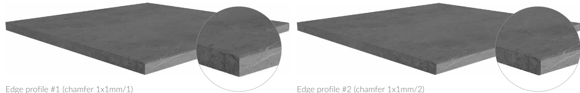
Edge profile #1 (chamfer 1x1mm/1) Kantenprofil #1 (Abschrägung 1x1mm/1)
