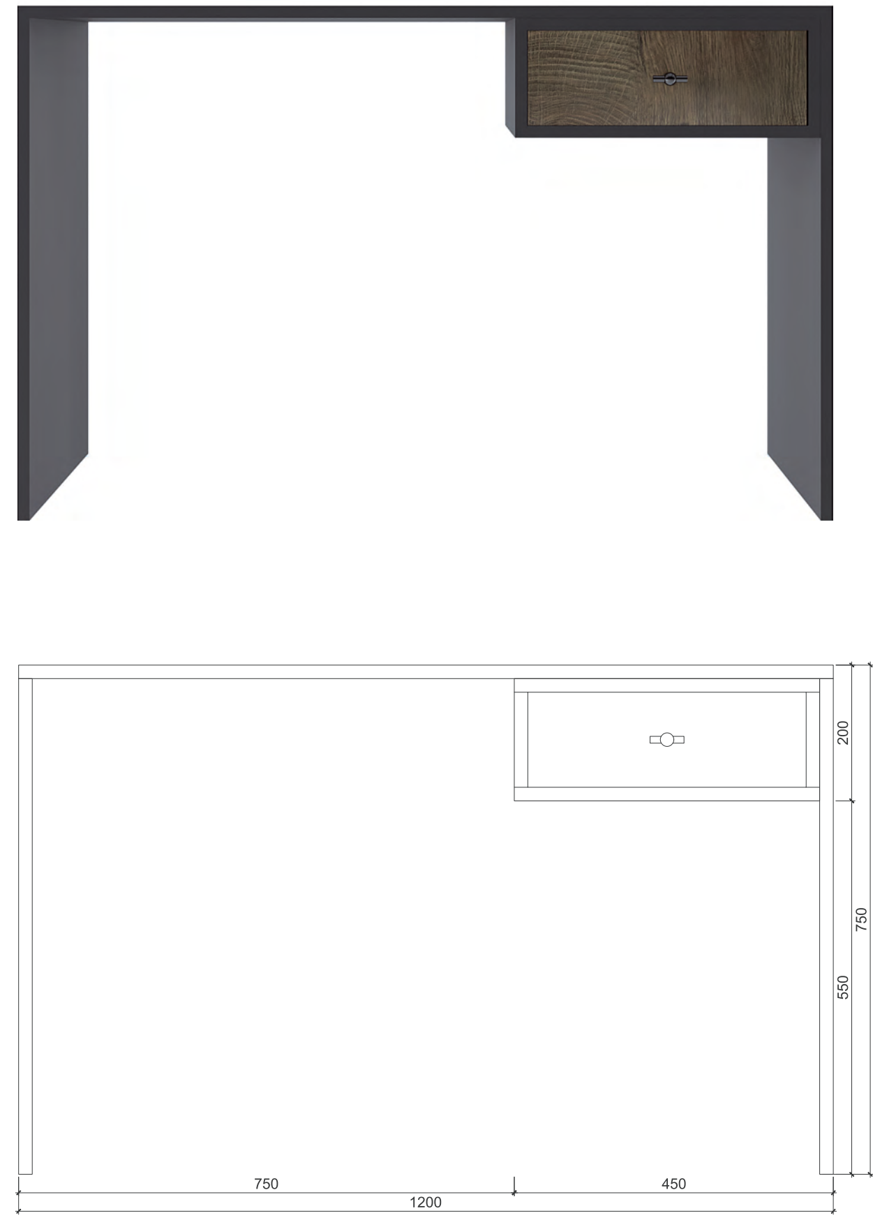
Рабочий стол Work desk
