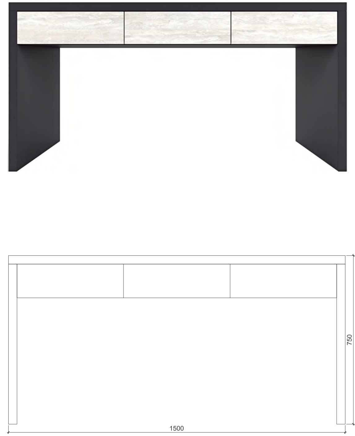
Рабочий стол Work desk
