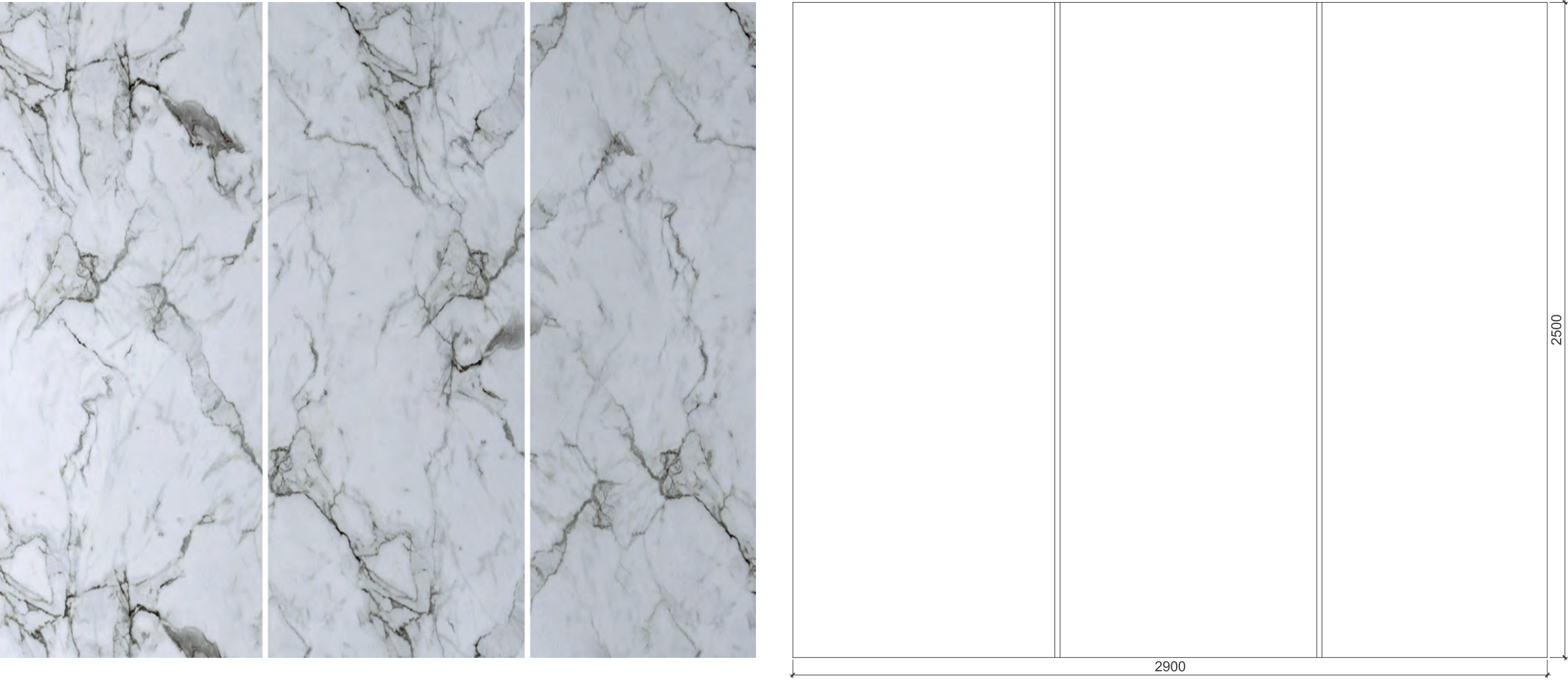
Стеновая панель за кроватью (МДФ/НПЛ 7мм) Wall panel behind the bed (MDF/HPL 7mm)
