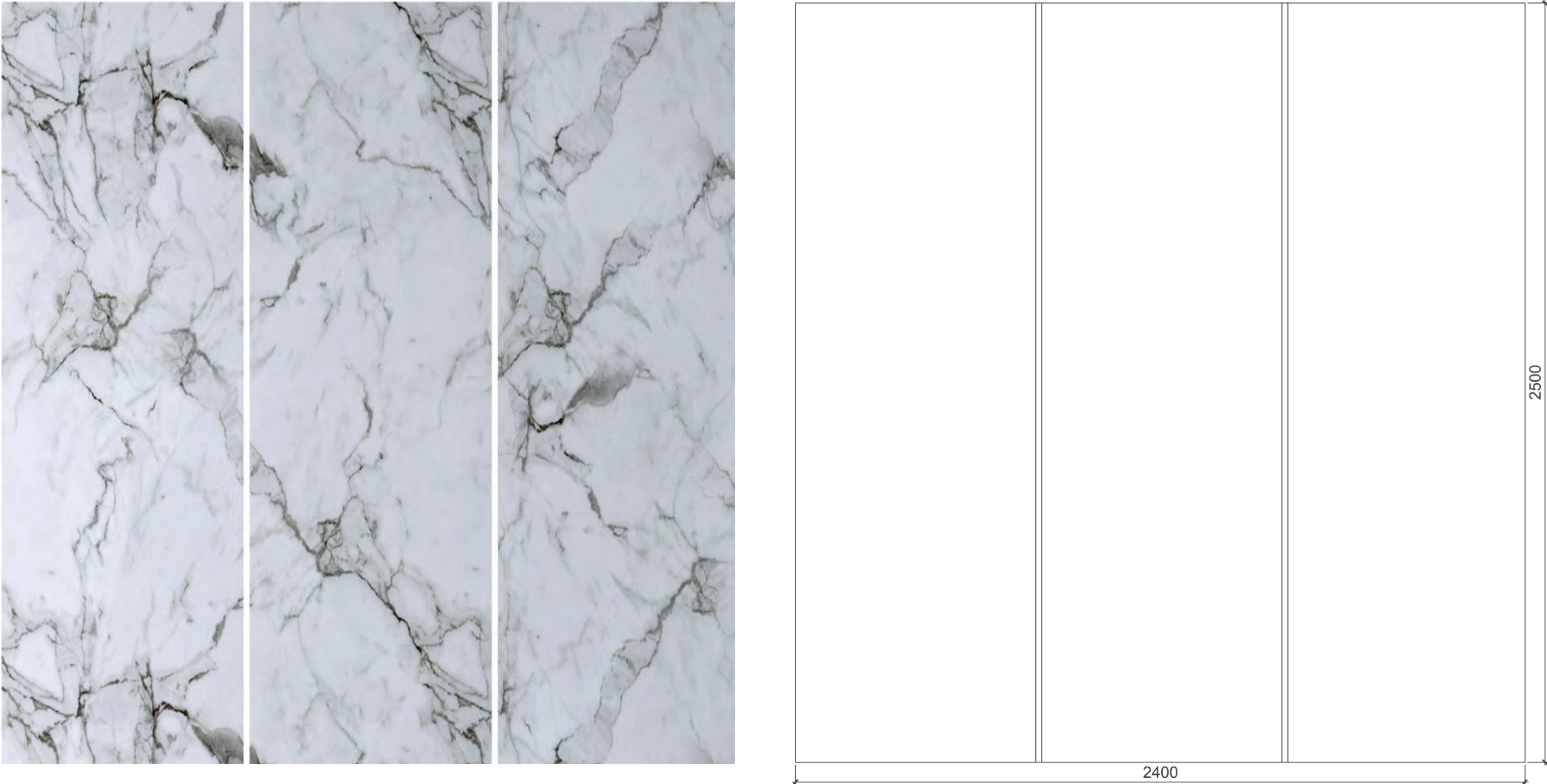
Стеновая панель за ТВ (МДФ/НПЛ 7мм) Wall panel behind the TV (MDF/HPL 7mm)
