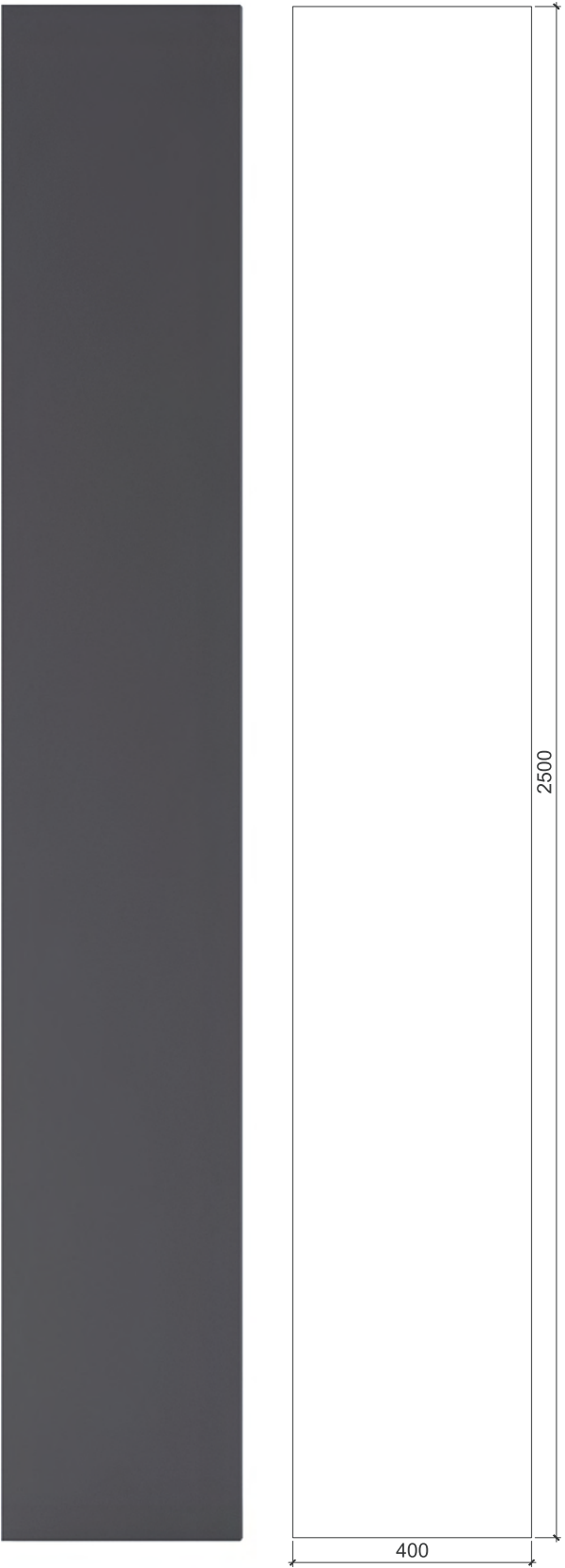
Стеновая панель (ЛДСП 18мм) Wall panel (MFC 18mm)
